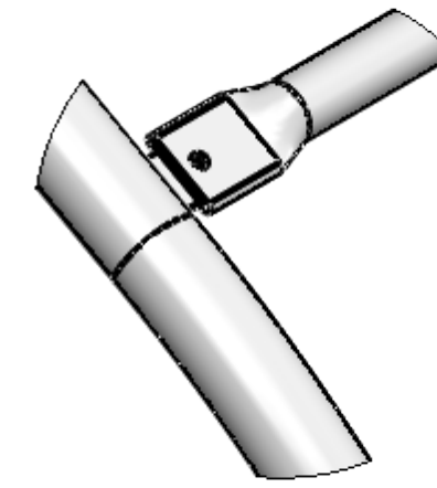
DETAIL E MÉRITKO 1 : 5
