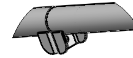
DETAIL C MÉRITKO 1 : 5
